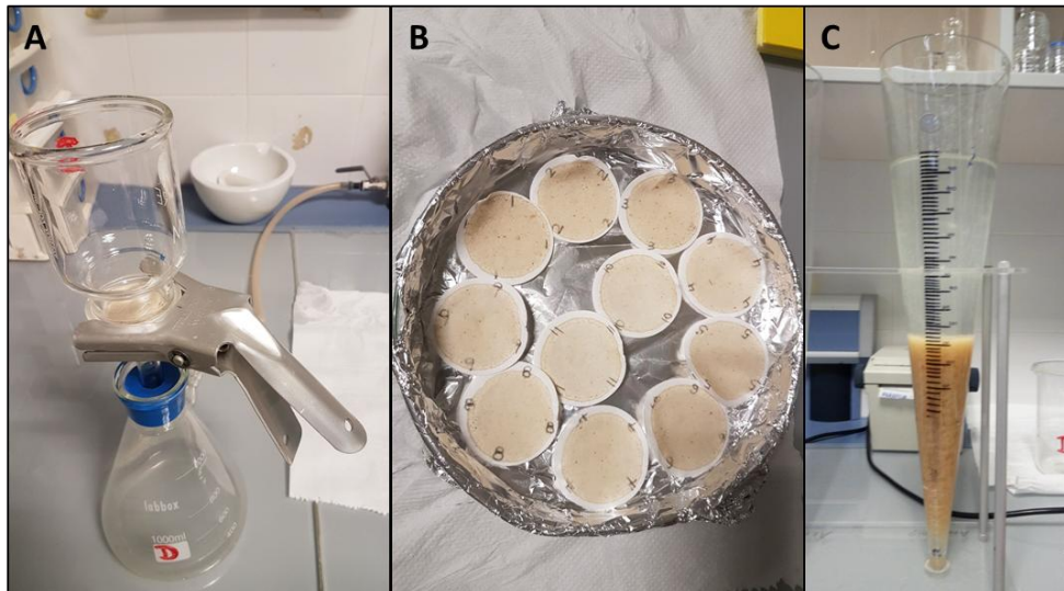
Figura 2. A) Montaje experimental para la filtración de sólidos suspendidos. B) Filtros con los sólidos suspendidos resultantes del proceso de filtración. C) Determinación de IVL en un cono Imhoff.
